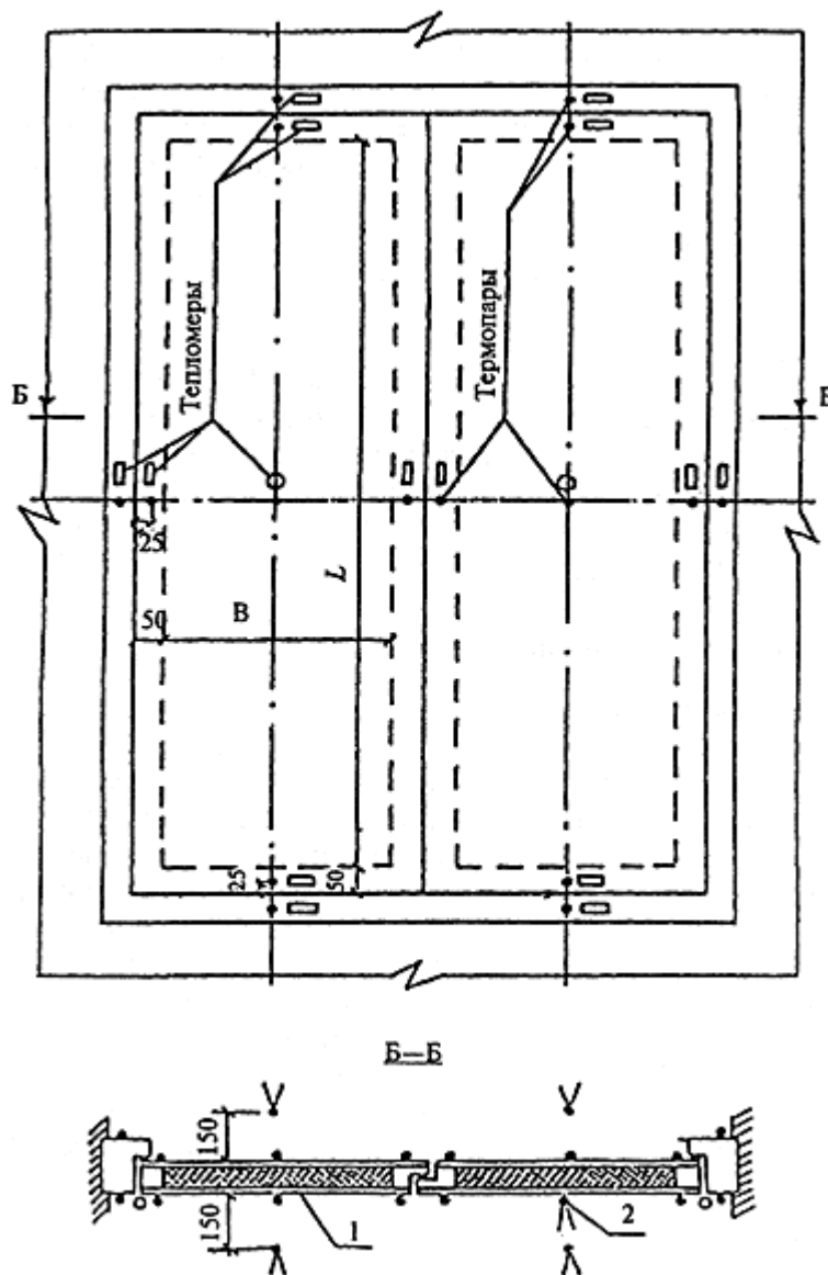
1 - испытываемый образец; 2 - рабочий спай термодатчика
