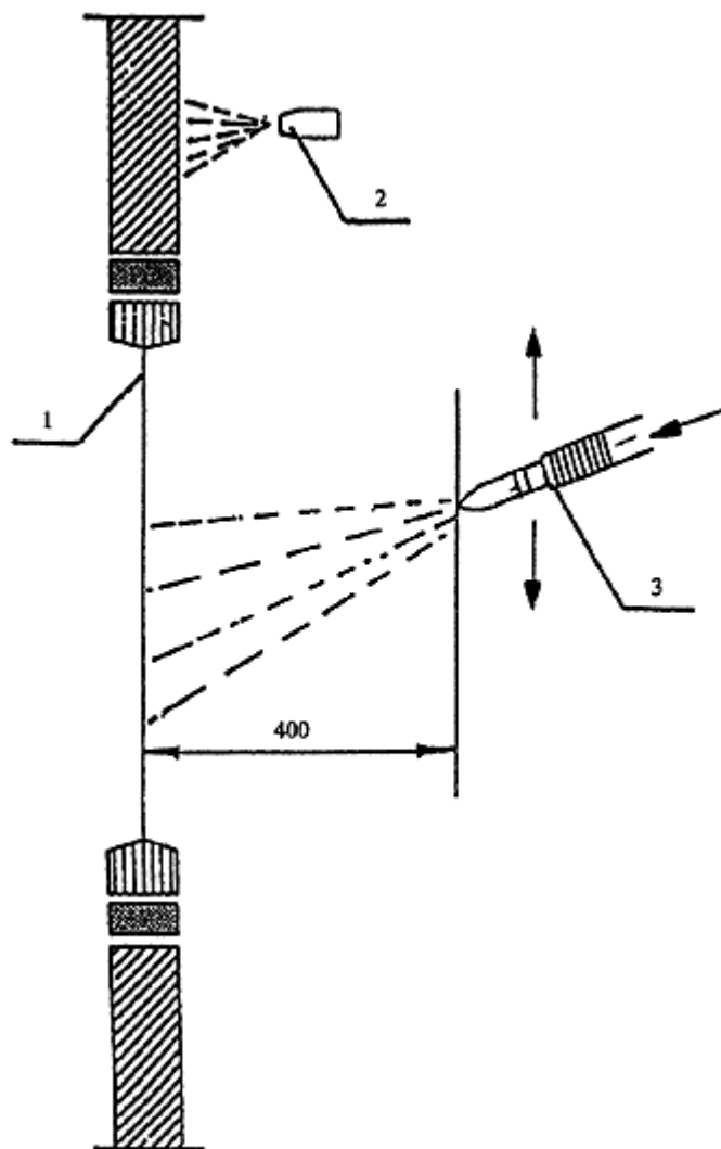
1 - образец; 2 - форсунка верхнего неподвижного ряда; 3 - подвижная форсунка
