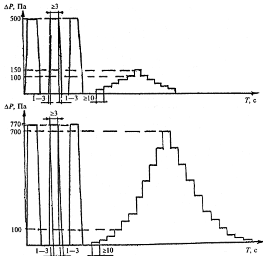
Рисунок 2 - Примеры построения графиков испытаний при контрольном конечном давлении 150 и 700 Па
